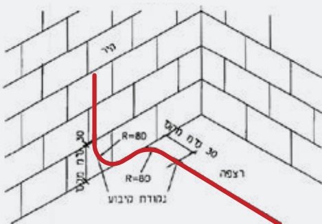
D - הקוטר החיצוני של הצינור המתעקל R - רדיוס כיפוף הצינור
